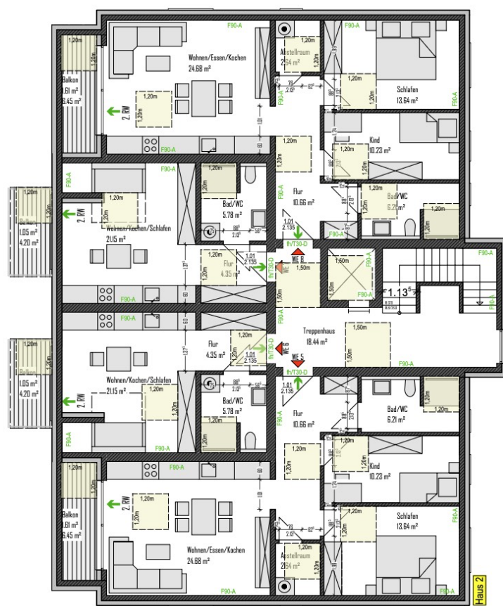
1.OG
