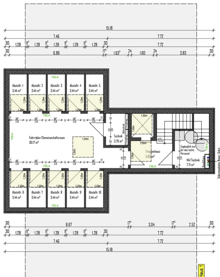
Keller
