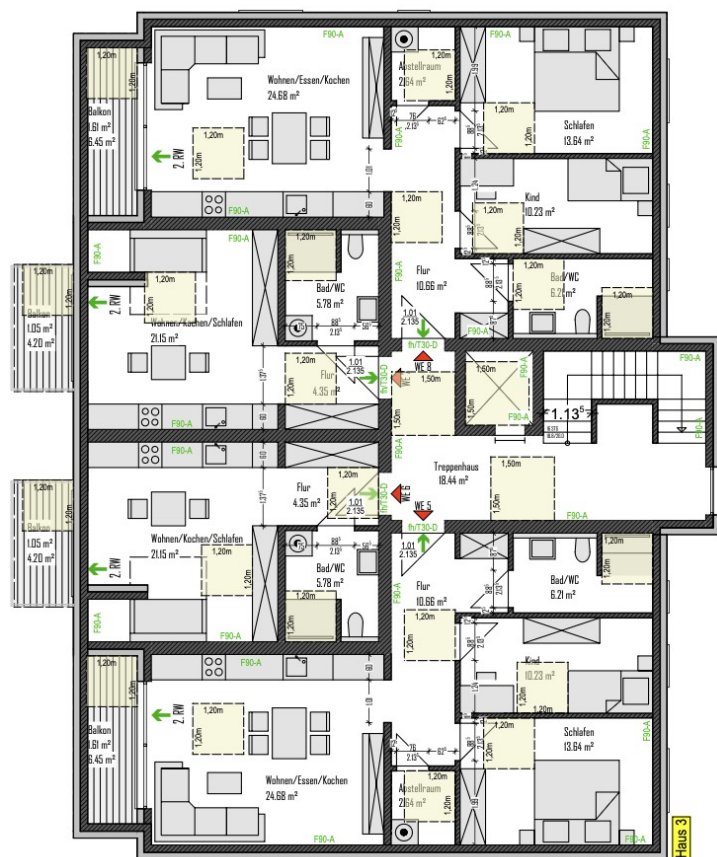
1.OG
